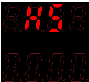
互锁信号输入停机代码 (外部输入应急互锁信号)
